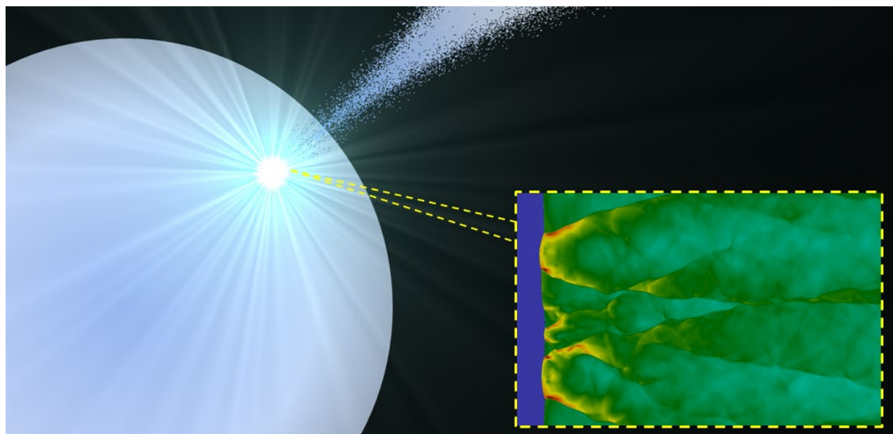
白色矮星表面への質量降着流により発生する、Ia 型超新星の第一段階のデトネーションのイメージ。右のセル構造の拡大図は、本研究グループによる数値シミュレーション結果を示す(Credit: 岩田、前田)
