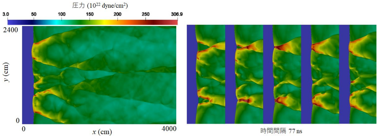
図1 セル構造シミュレーション結果の例。密度 1 \times 10^6 g/cm 3 、ヘリウム質量分率 0.6 における圧力分布：(左)計算領域全体の瞬間図 (右)77ns 間隔の連続図
