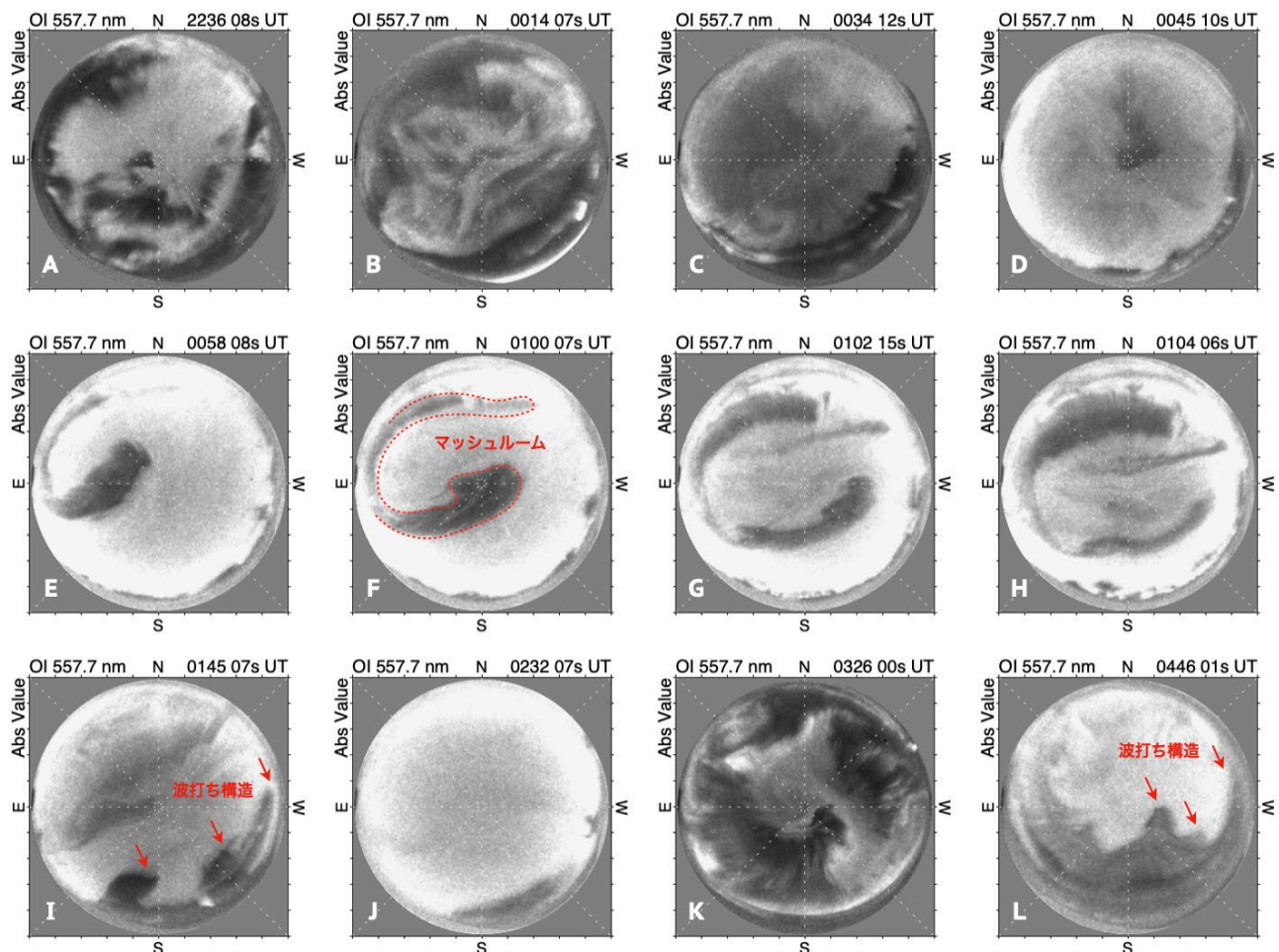
図 3: 電子の雨に伴って発生したポーラーレイオーロラが最も明るくなった時間帯に得られた地上からのオーロラ撮像データ。557.7 nm の緑色の発光を観測するカメラによって得られたデータを示しています。オーロラの形態に特徴的な模様（マッシュルームのような形や波打ち構造）が見られることが分かります。
