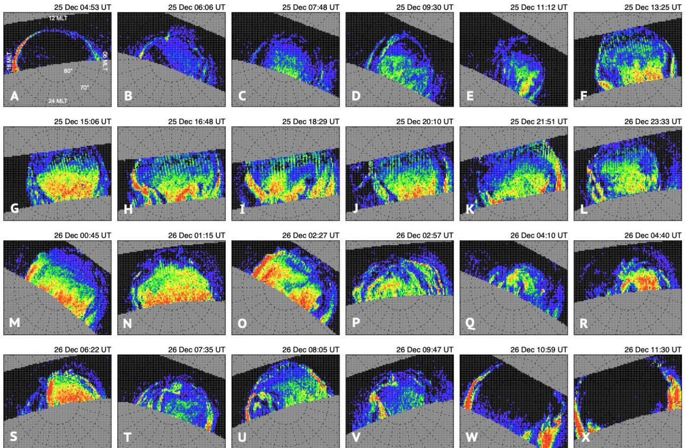
図 1: DMSP 衛星に搭載された紫外線撮像装置によって得られた北極域のオーロラの広域分布。2022 年 12 月 25 日の世界時 4 時 53 分から翌日の世界時 11 時 30 分までの 24 枚の連続画像。画像の中央が磁気的な北極点、上側が太陽方向になっています。磁気的な極を取り囲む約数千 km 四方の領域（極冠域）が、明るいオーロラによって覆われていることが分かります。
