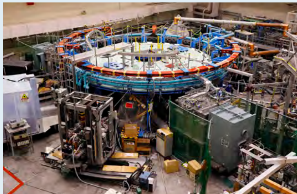
数千万度の超高温プラズマを発生させる京大独自の「ヘリオトロン」装置。
